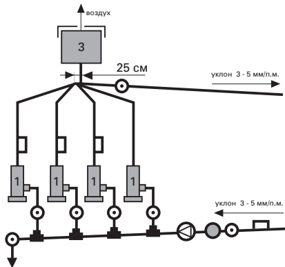
Рис. 2 Параллельное подключение.
